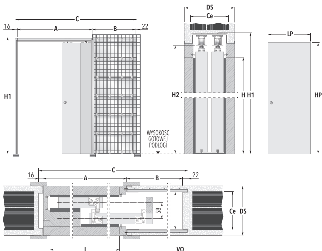
WYMIARY KASETY STANDARDOWEJ
