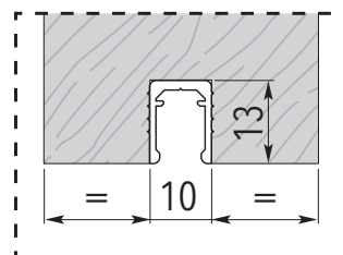
Wymiar frezu pod profil aluminiowy
